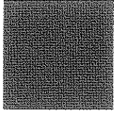
正方形
