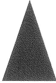
三角形
