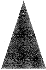
三角形
